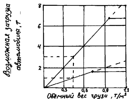
Рис. 20 – График определения загрузки автомобиля
