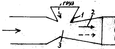
Рис. 22 - Принцип работы инжекторного загрузочного устройства
