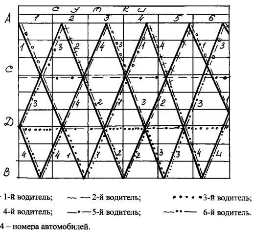
Рис.36 -График оборота автомобилей при сменно-групповой езде
