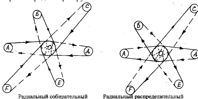
Рис. 28 - Схемы радиальных маршрутов
