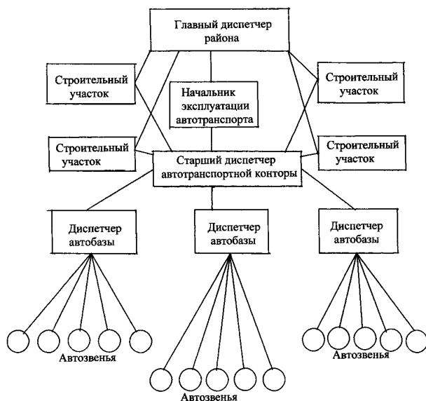
Рис.43 - Схема централизованного управления перевозками на крупном строительстве
