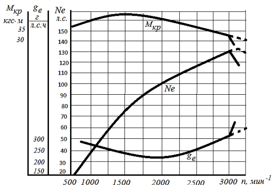
Рис. 49 - Скоростная характеристика двигателя
