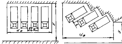
Рис. 14 – Торцевое (а) и косоугольное (б) расположение автомобилей
