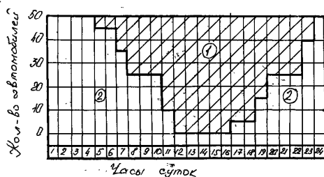
Рис.44 - Ступенчатый график выпуска автомобилей на линию:
