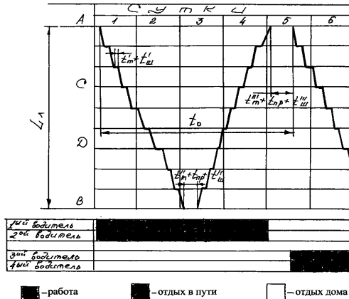
Рис.34 - График оборота транспортного средства к работе водителя при турной езде
