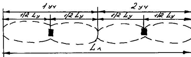
Рис.40 - Схема участкового движения с длинными участками
