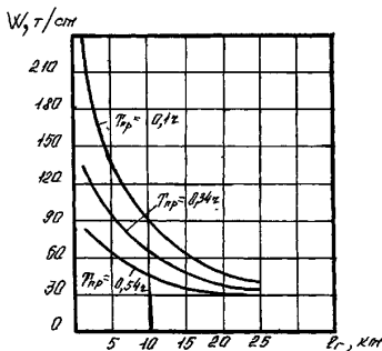
Рис.18 -Влияние времени простоя под погрузкой и разгрузкой на производительность
