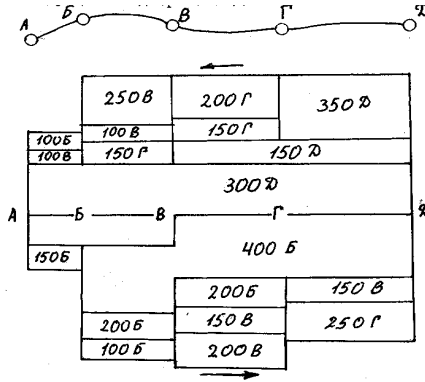
Рис. 6 - Схема расположения грузообразующих и грузопоглощающих пунктов и эпюра грузопотоков.
