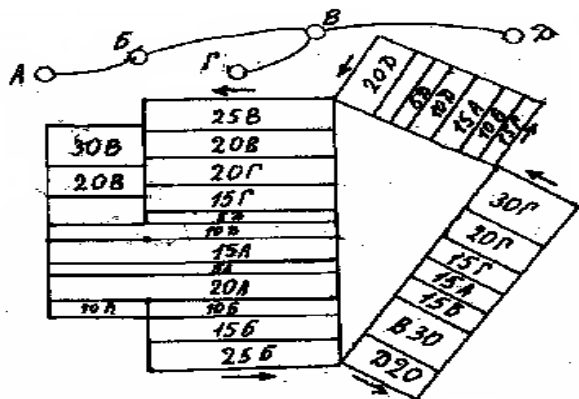
Рис. 7 - Расположение грузообразующих и грузопоглощающих пунктов и эпюра грузопотоков
