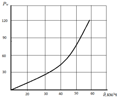
Рис. 46 - График зависимости силы сопротивления ветровых и воздушных воздействий от скорости движения автомобиля
