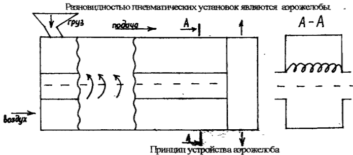
Рис. 23 – Схема аэрожелоба
