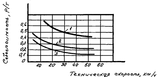
Рис. 21 - Зависимость себестоимости транспортирования от изменения технической скорости автомобилей:
