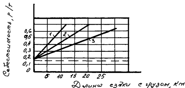
Рис. 22 - Зависимость себестоимости транспортирования от изменения длины ездки автомобилей с грузом:
