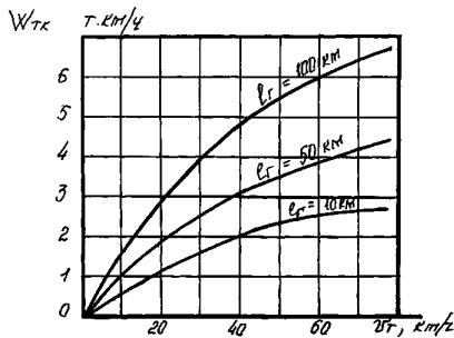
Рис. 16 - Влияние средней технической скорости на производительность
