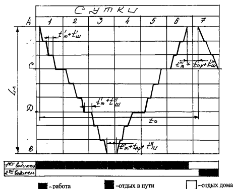
Рис.33 - График оборота транспортного средства и работы водителя при одиночной езде
