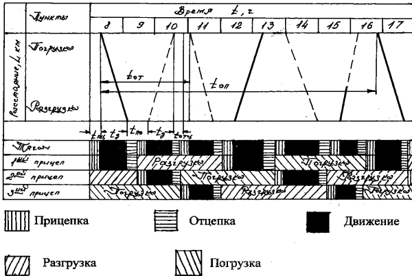
Рис. 30 - График работы одного автомобиля-тягача с тремя полуприцепами:
