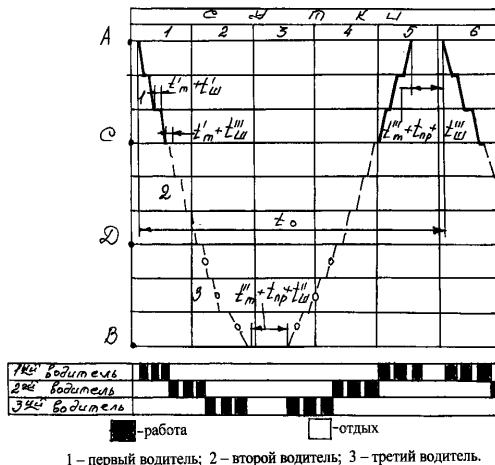
Рис.35 - График оборота транспортного средства и работы водителей при сменной езде
