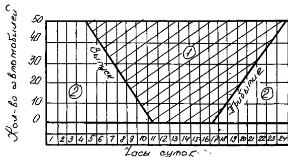
Рис.45 - График выпуска автомобилей цепочкой на линию
