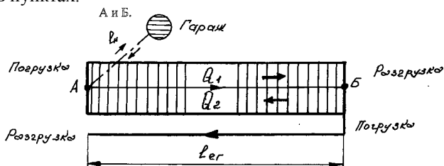
Рис. 25 - Схема маятникового маршрута с гружеными пробегами в обоих направлениях Q_1 и Q_2 - грузовые потоки.
