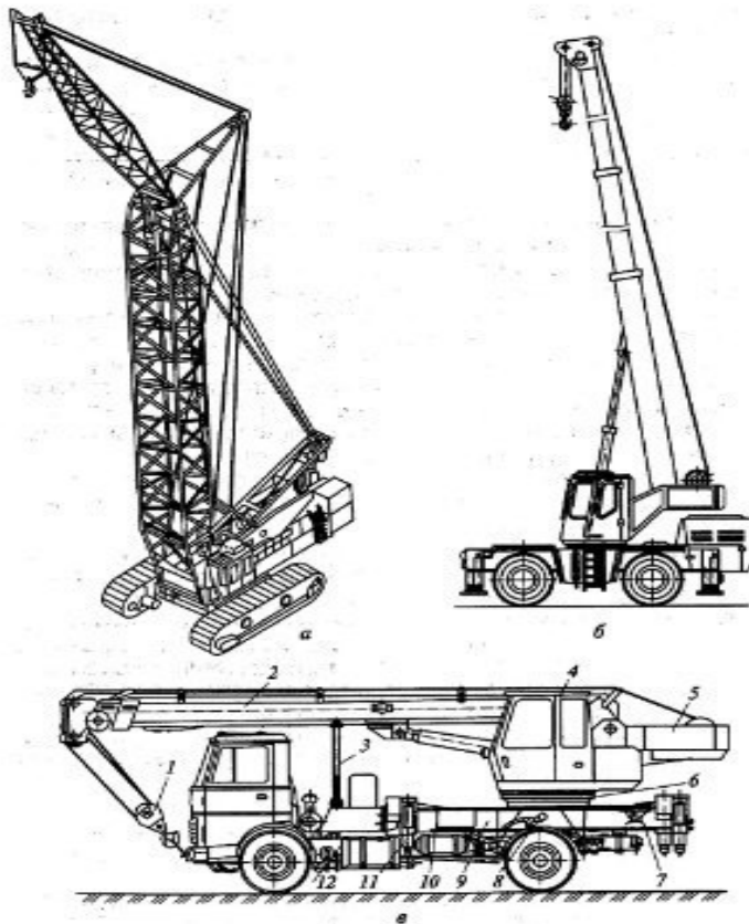
Рис. 29 - Стреловые самоходные краны:
