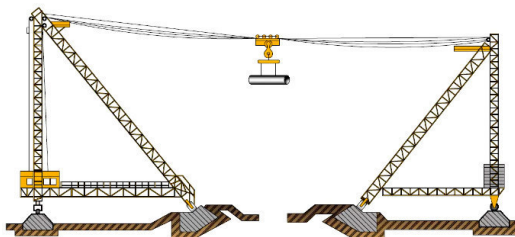
Рис. 27 - Кабельный кран
