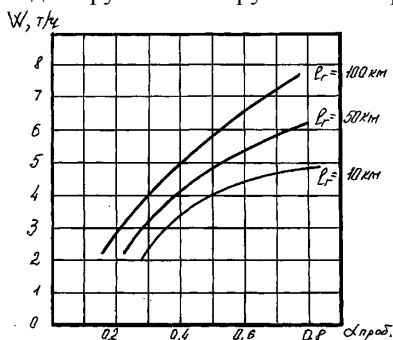
Рис. 17 - Влияние коэффициента использования пробега на производительность
