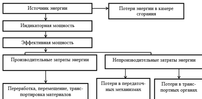
Рис. 47 - Схема распределения энергии
