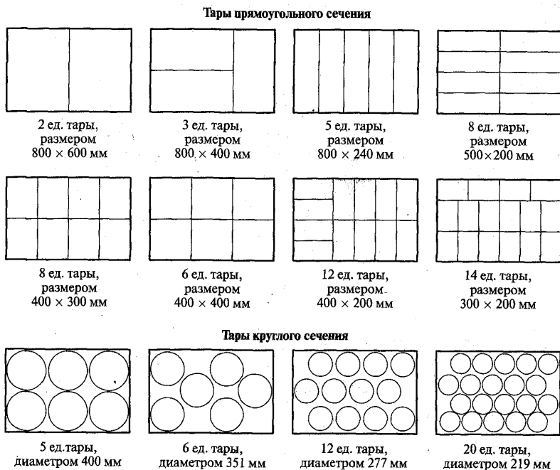
Рис. 3 - Примеры размещения транспортной тары различного размера на поддоне 1200 х 800 мм
