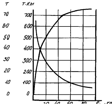
Рис. 15 - Влияние расстояния перевозок груза на производительность транспортного агрегата
