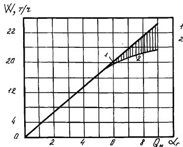
Рис.19- Влияние коэффициента грузоподъемности на производительность:
