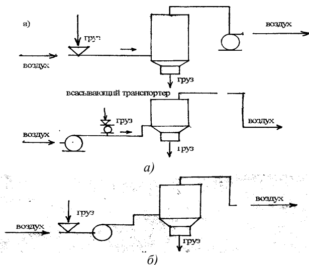
Рис. 21 – Типы пневмотранспортеров:
