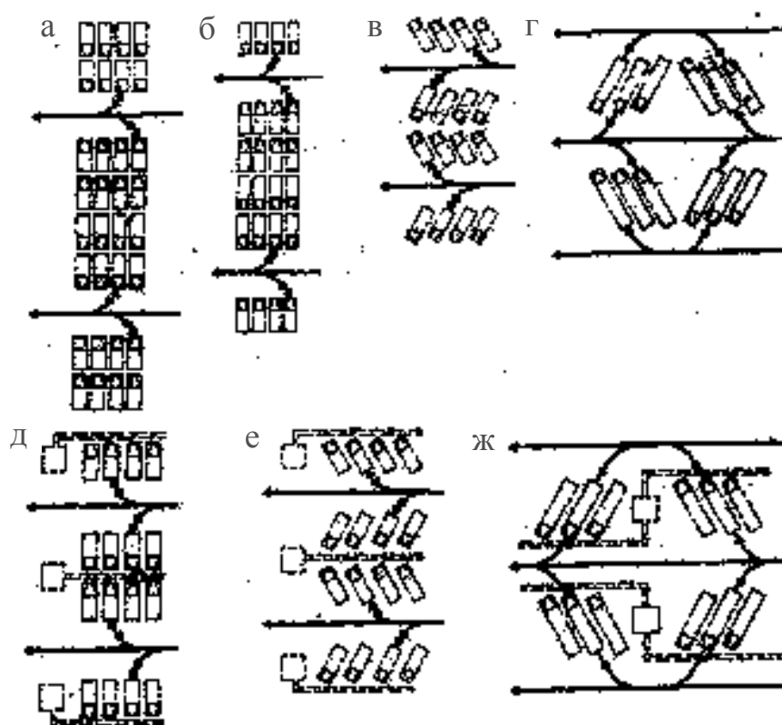
Рисунок 2.1 - Схема расстановки подвижного состава на открытых площадках хранения
