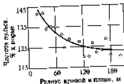
Рис. 5.16. Зависимость частоты пульса водителя от радиуса кривой в плане
