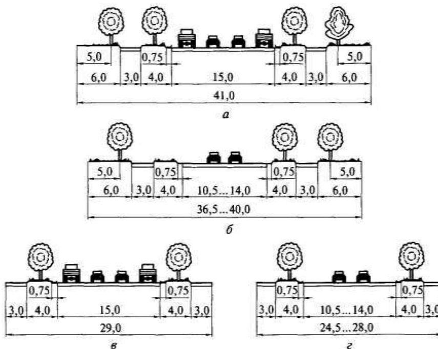
Рис. 1.8. Поперечные профили магистральных улиц районного значения (а, в) и жилых улиц (б, г):
