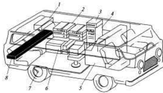
Рис. 8.7. Ходовая психофизиологическая лаборатория:
