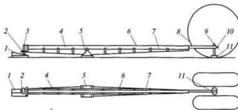
Рис. 3.6. Длиннобазовый рычажный прогибомер:
