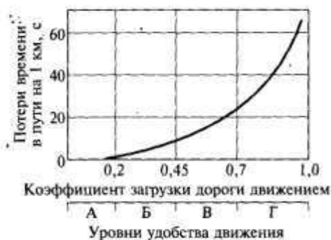
Рис. 5.5. Потери времени в пути на автомобильной магистрали с четырьмя полосами при разных уровнях удобства движения
