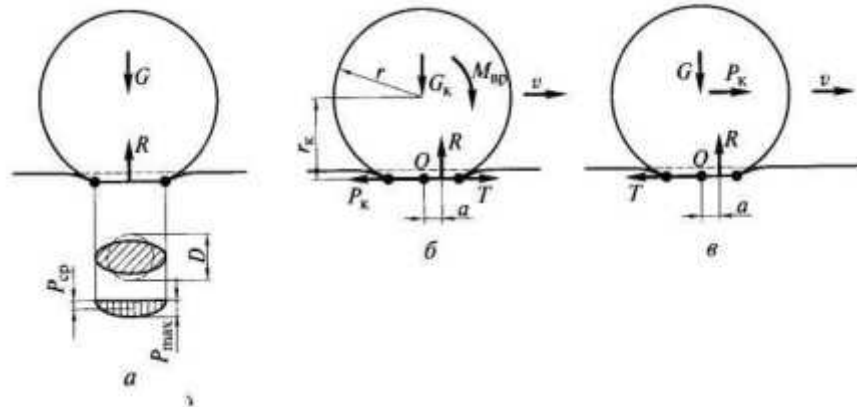
Рис. 3.1. Схема сил, действующих на дорожное покрытие:
