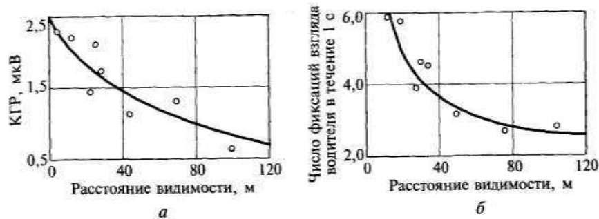
Рис. 5.17. Влияние расстояния видимости на кривых в плане горных дорог ( R = 50 \dots 100 м) на психофизиологические показатели водителя: а - изменение кожно-гальванической реакции (КГР); б - изменение числа фиксаций взгляда водителей в секунду
