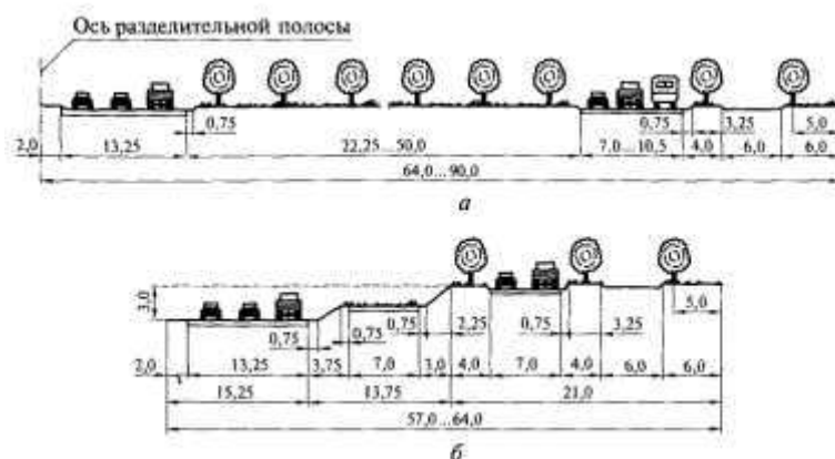
Рис. 1.6. Поперечные профили городских скоростных дорог (размеры даны в метрах): a - в одном уровне; б - в выемке
