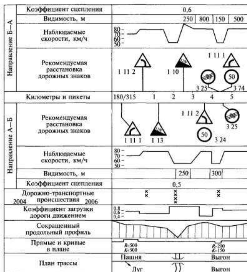
Рис. 7.8. Схема расстановки дорожных знаков
