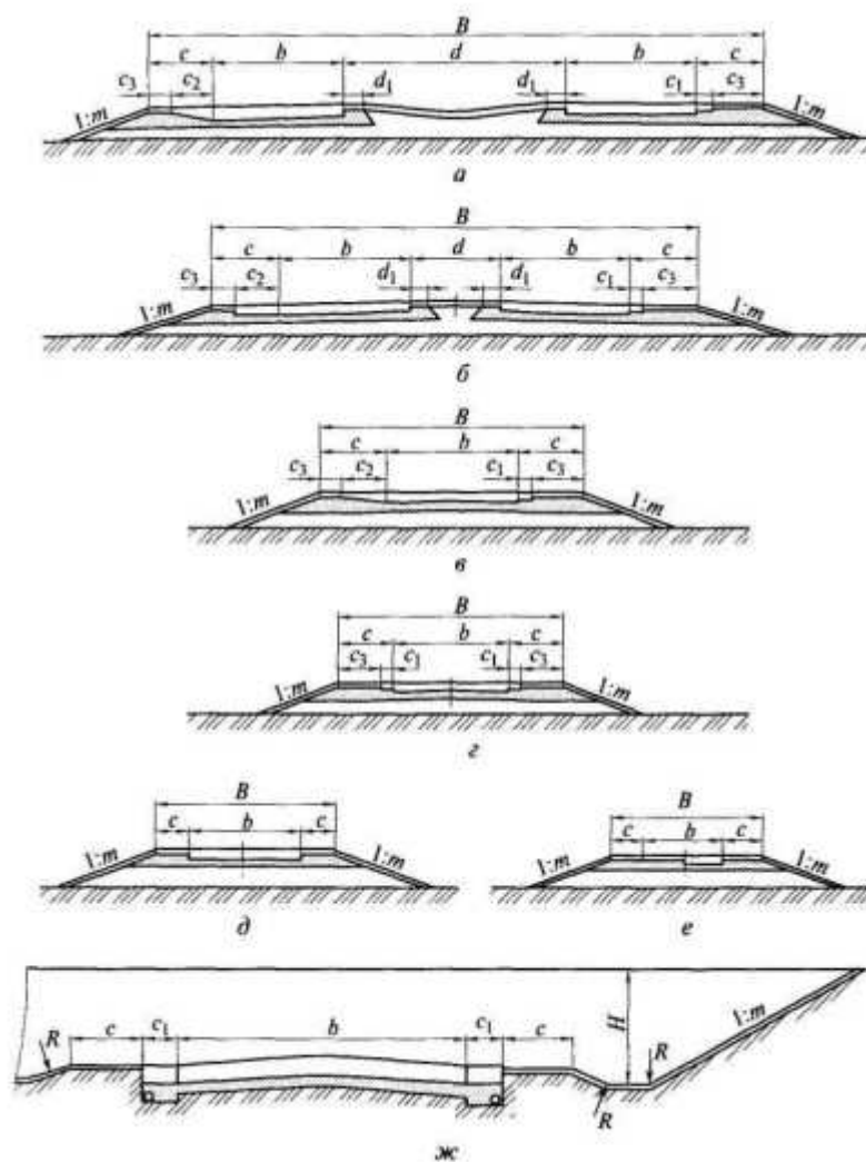
Рис. 1.9. Типовые поперечные профили земляного полотна: a, б - дорог I категории; в, г - дорог II категории; д - дорог III, IV категории; е - дорог V категории; ж - дорог в выемке; B - ширина земляного полотна; b - ширина проезжей части; d - ширина разделительной полосы; d 1 - ширина укрепления; c - ширина обочины; c 1 - ширина дренажа; c 2 - ширина укрепительной полосы; c 3 - ширина укрепленной обочины; 1 : m - уклон откоса; H - глубина выемки; R - радиус
