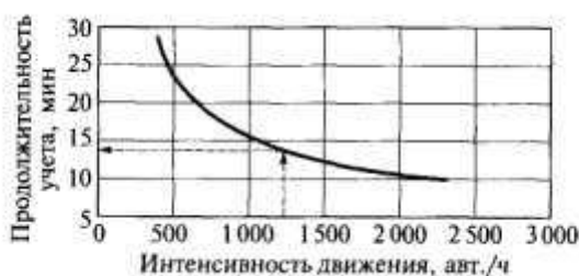
Рис. 8.1. График для определения продолжительности учета часовой интенсивности движения с точностью 10 %
