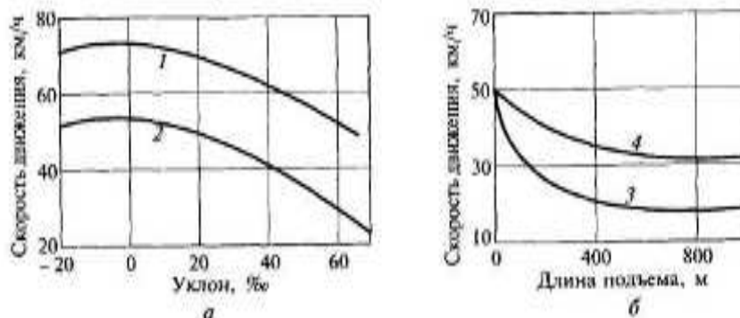
Рис. 5.13. Влияние уклона (а) и длины подъема (б) на скорость движения: а - влияние уклона; б - влияние длины подъема; 1 - легковые автомобили; 2 - грузовые автомобили; 3 - i = 70 ‰; 4 - i = 50 ‰
