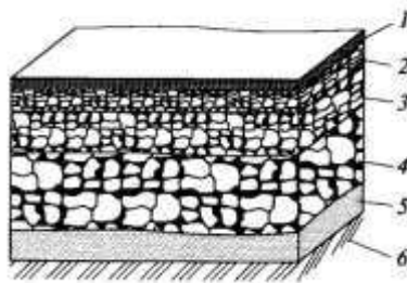
Рис. 1.10. Дорожная одежда:
