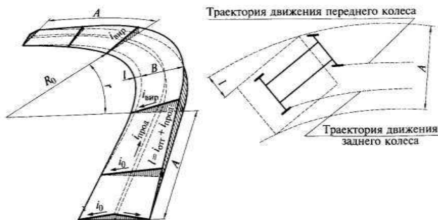
Рис. 1.1. Схема виража:
