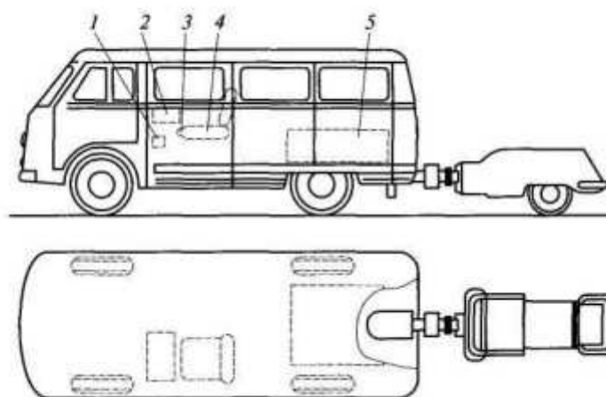
Рис. 4.6. Динамометрическая установка ПКРС-2:
