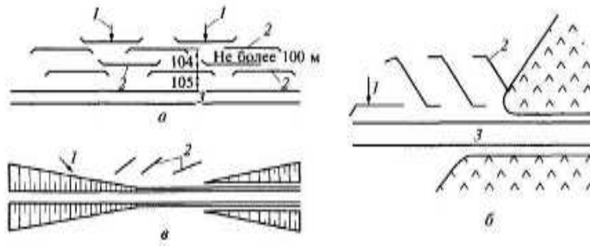
Рис. 12.1. Расположение снегозадерживающих заборов по отношению к автомобильной дороге:
