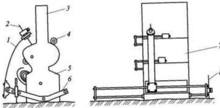
Рис. 4.21. Профилограф Союздорнии:
