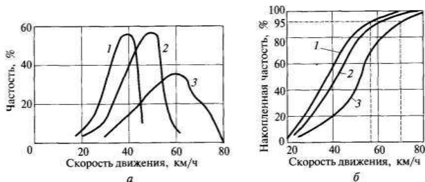
Рис. 5.7. Обработка данных наблюдений методами математической статистики: a - кривые распределения; б - кумулятивные кривые; 1 - интенсивность движения 400 авт./ч; 2 - интенсивность движения 400 авт./ч (в потоке на 10 % меньше грузовых автомобилей); 3 - интенсивность движения 150 авт./ч
