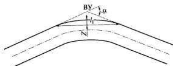
Рис. 7.3. Схема для определения радиуса кривой по хорде: l_1 - хорда; Z - отрезок; остальные обозначения см. на рис. 7.2
