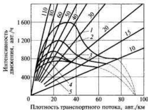
Рис. 4.25. Основная диаграмма транспортного потока для реальных условий движения:
