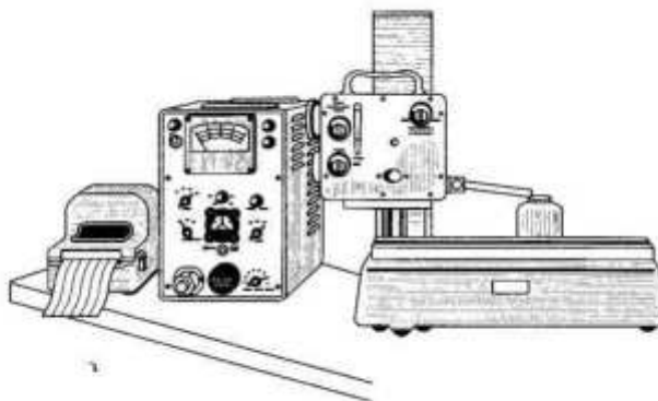
Рис. 4.22. Индуктивный профилограф МАДИ
