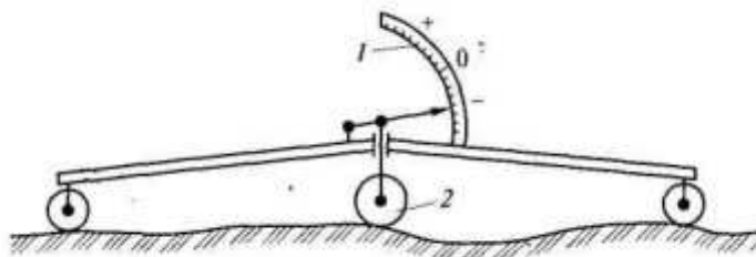
Рис. 4.3. Передвижная двухопорная рейка ПКР-1: 1 - шкала замера неровностей; 2 - колесо-индикатор
