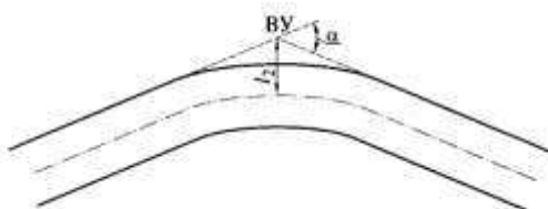
Рис. 7.4. Схема для определения радиуса кривой по биссектрисе: l_2 - длина отрезка биссектрисы от вершины угла до середины проезжей части; остальные обозначения см. на рис. 7.2
