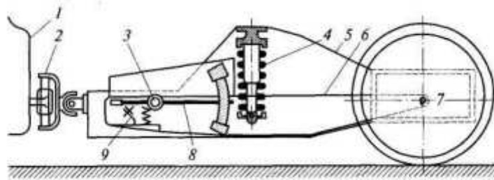
Рис. 4.9. Схема прибора для записи микропрофиля конструкции МАДИ:
