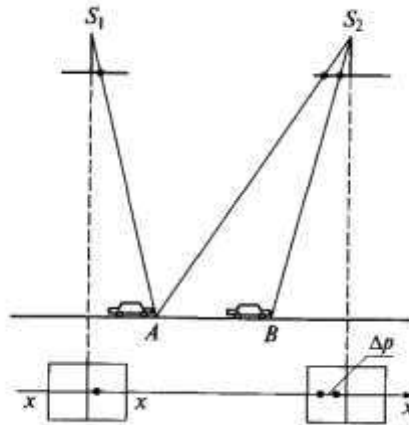
Рис. 8.10. Определение скорости движения автомобиля по способу псевдопараллакса:
