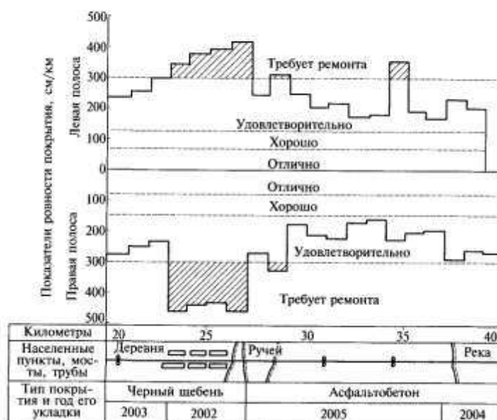
Рис. 7.6. Линейный график измерения ровности дорожного покрытия
