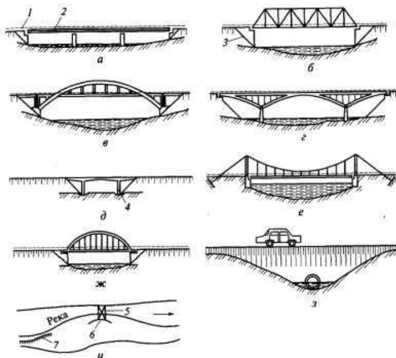
Рис. 1.14. Искусственные сооружения на автомобильных дорогах:
