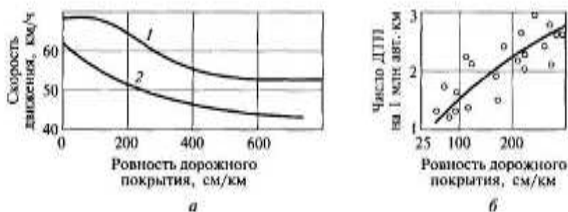
Рис. 4.12. Влияние ровности дорожного покрытия на скорость движения (а) и аварийность (б):
