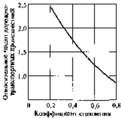
Рис. 4.14. Влияние коэффициента сцепления на аварийность
