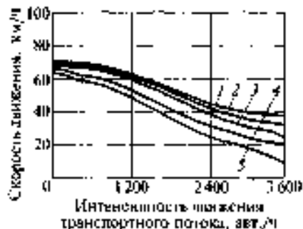
Рис. 5.12. Зависимость скорости движения от интенсивности движения транспортного потока на четырехполосной автомагистрали при расстоянии между автобусными остановками 500...1000 м (2, 4) и до 500 м (3, 5):
