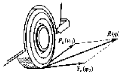
Рис. 3.2. Силы, действующие на дорожное покрытие на криволинейных участках:
