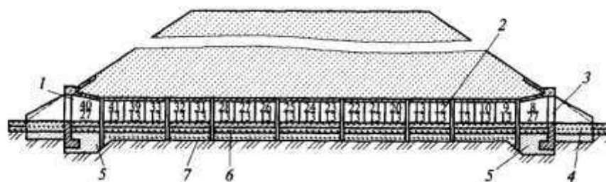
Рис. 1.13. Водопрopusкная труба:
