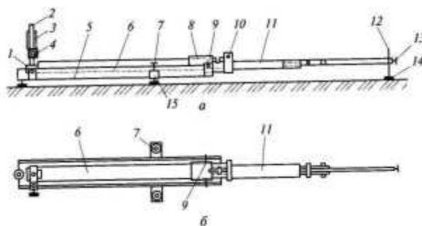
Рис. 3.5. Рычажный прогибомер МАДИ - ЦНИЛ:
