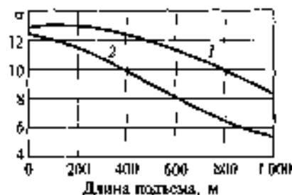
Рис. 5.14. Зависимость среднего квадратического отклонения скоростей движения от длины подъема:
