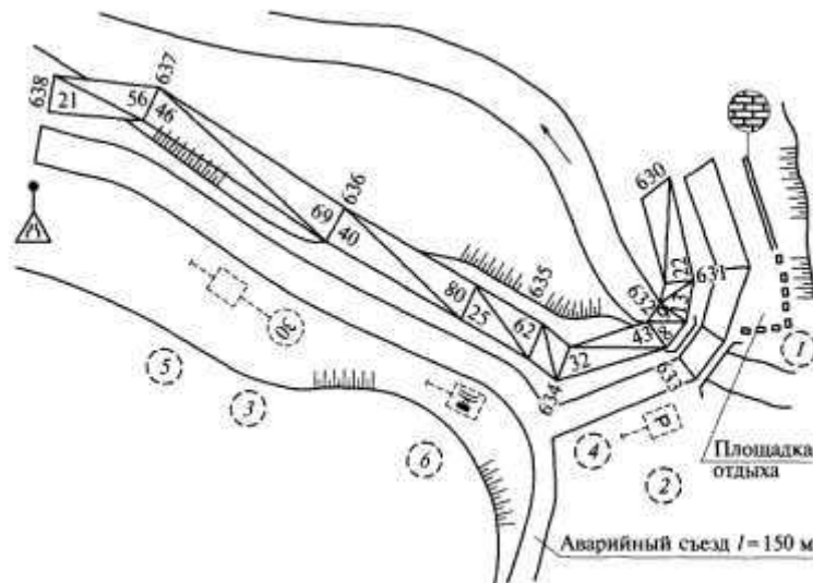
Рис. 7.9. Общий вид одного листа альбома комплексного инженерного обустройства горной дороги (пунктиром показаны намечаемые мероприятия):
