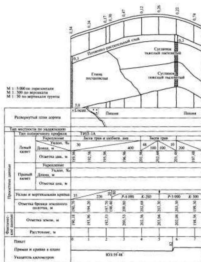
Рис. 1.3. Продольный профиль автомобильной дороги
