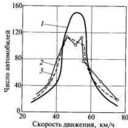
Рис. 5.9. Кривые распределения скоростей движения: 1 - рассчитанная по формуле (5.4); 2 - рассчитанная по формуле (5.5); 3 - фактическая кривая
