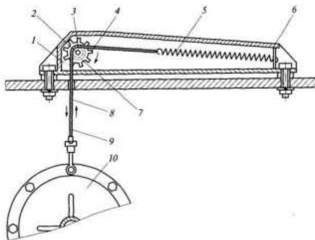
Рис. 4.7. Толчкомер ТЭД-2М:
