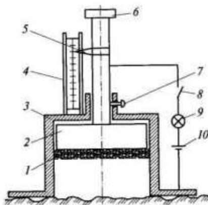
Рис. 4.20. Магнитный прибор для измерения средней глубины впадин макрошероховатости дорожного покрытия:
