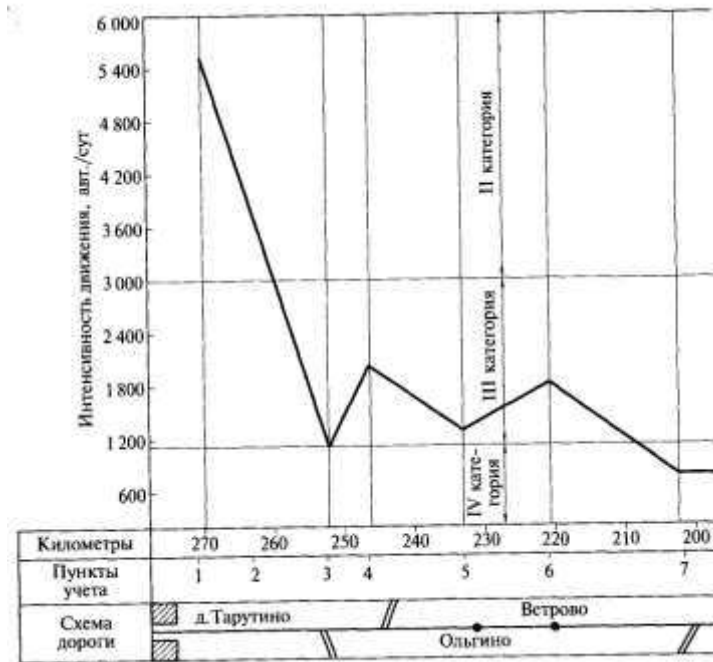
Рис. 8.3. Линейный график изменения интенсивности движения вдоль автомобильной дороги
