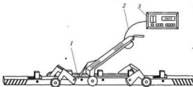
Рис. 4.4. Прибор РК-1:
