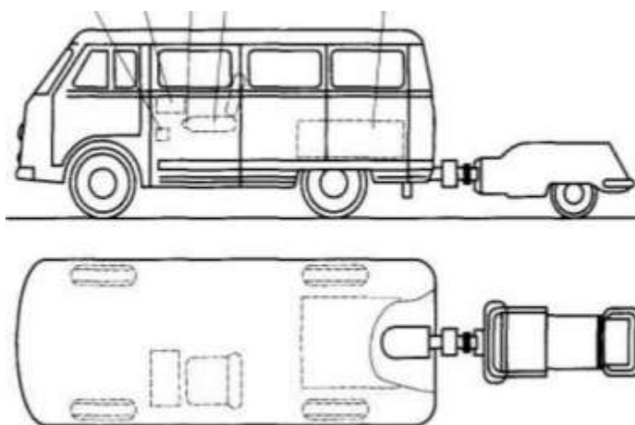
Рис. 4.6. Динамометрическая установка ПКРС-2: 1 - тормозная педаль прицепа; 2 - пульт управления; 3 - трос; 4 - место оператора; 5 - бак для воды 1 - кузов автомобиля, 2 - водораздатчик; 3 - трос; 4 - задний мост автомобиля
