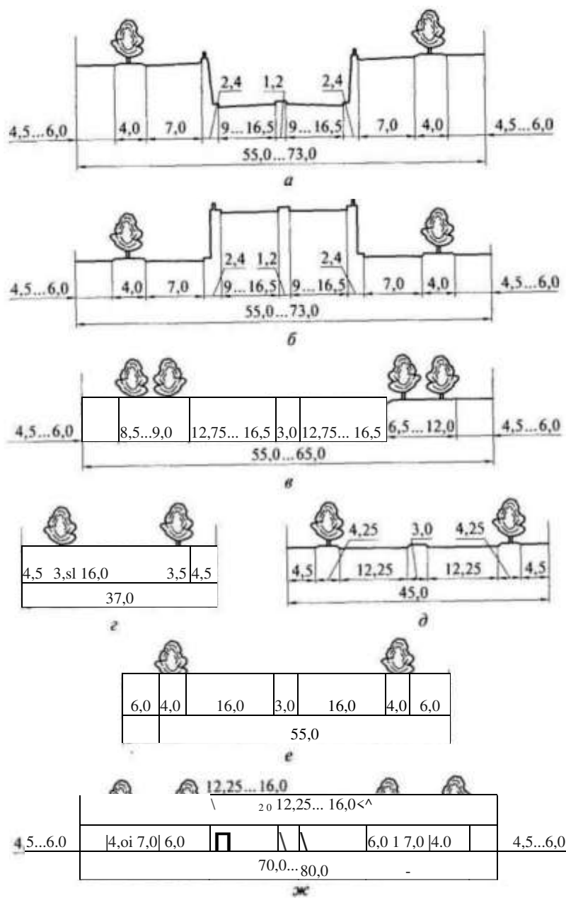
Рис. 1.7. Поперечные профили магистральных улиц общегородского значения с непрерывным движением ( а - в ) и с разными размерами движения ( г - ж ) (размеры даны в метрах): а - на подходах к тоннелям; б - на подходах к эстакадам; в - между пересечениями в разных уровнях; г, д, е - с небольшими, средними и значительными размерами движения соответственно; ж - с местными проездами
