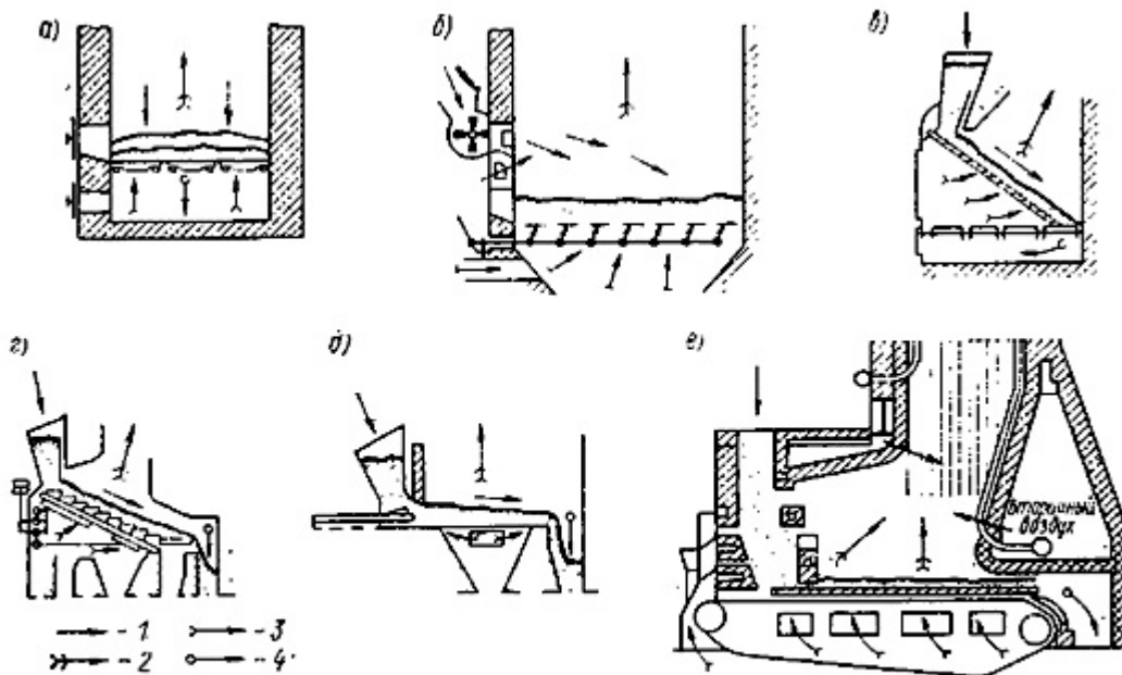
Рис. 15.2. Схемы слоевых топок
